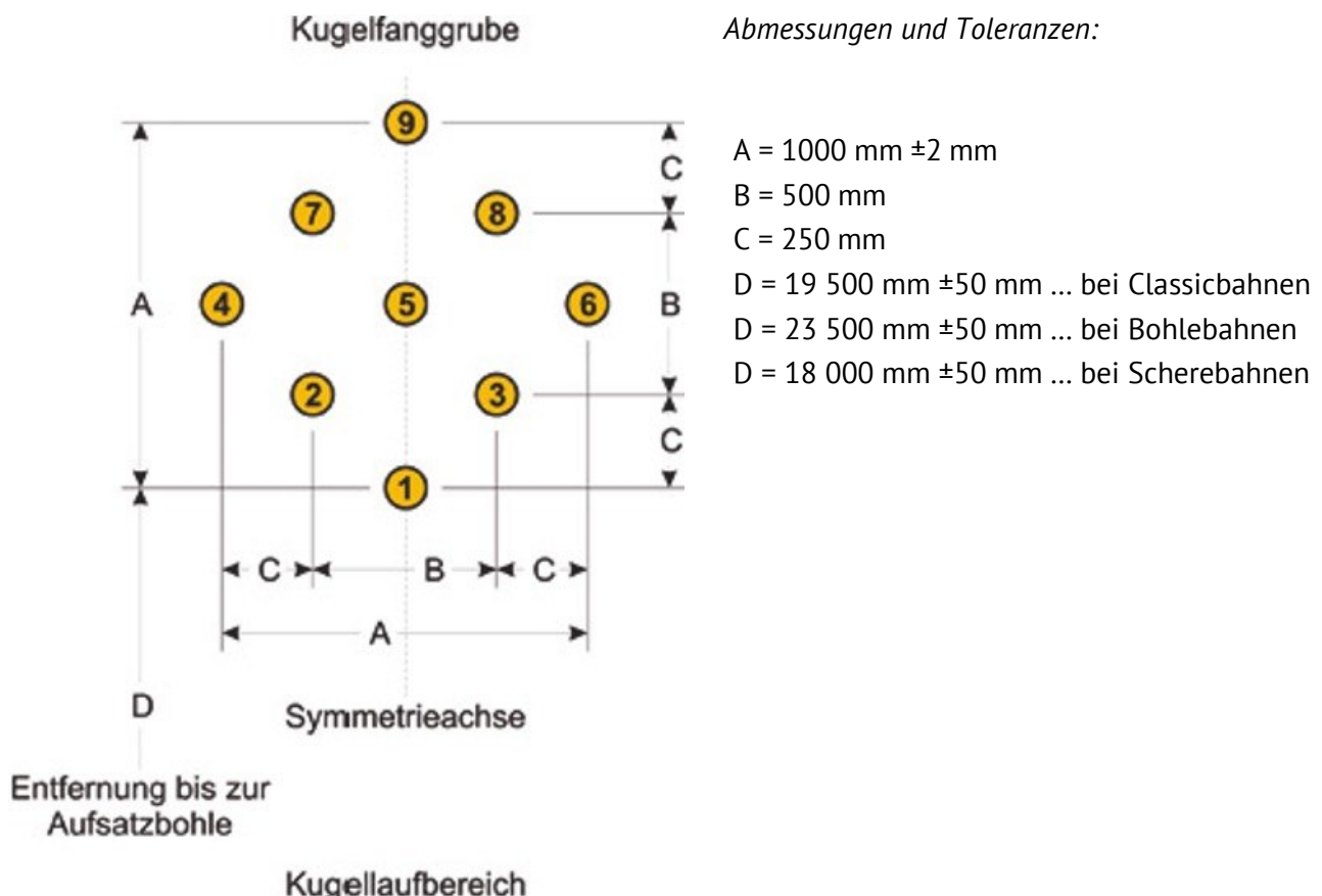
Abbildung 4 Anordnung und Bezeichnung der Kegel
