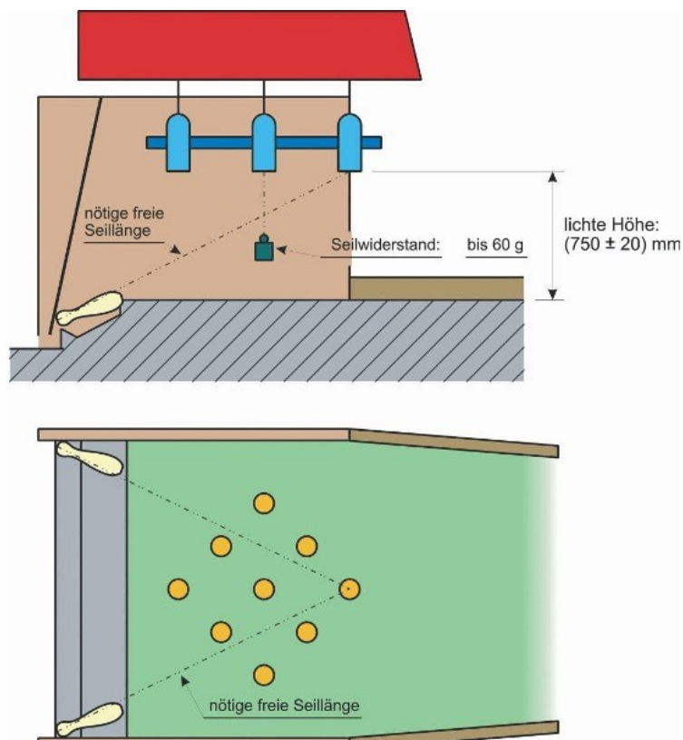
Abbildung 3 Anforderungen auf Kegelstellautomaten mit Seil
