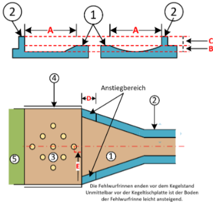
Abbildung 33: Ausführungsmöglichkeiten für Fehlwurfrinnen
