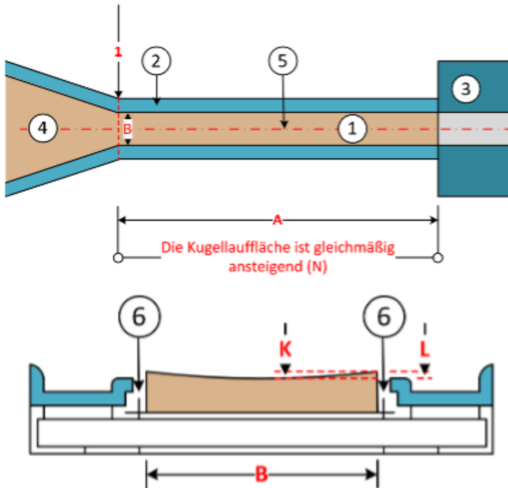
Abbildung 29 Gerader Teil der Kugellauffläche
