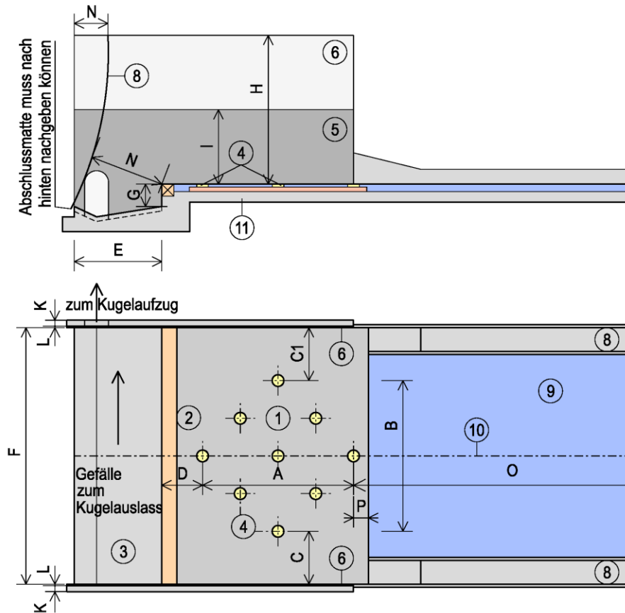
Abbildung 21 Der Kegelbereich bei Ausführung mit Kegeltischplatte und Fehlwurfrinnen
