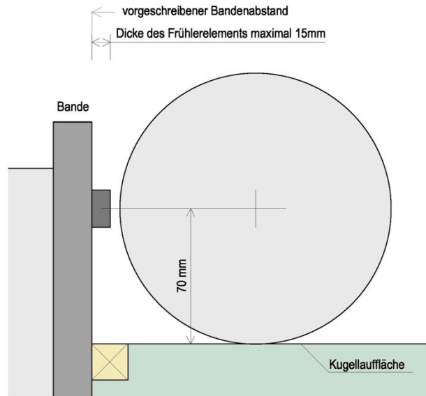
Abbildung 17 Fehlwurfanzeige
