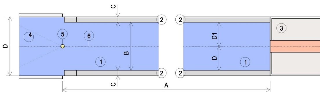
Abbildung 14 Kugelauffläche mit Fehlwurfrinnen
