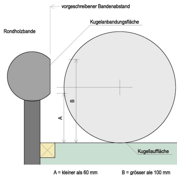
Abbildung 18 Banden aus Rundholz
