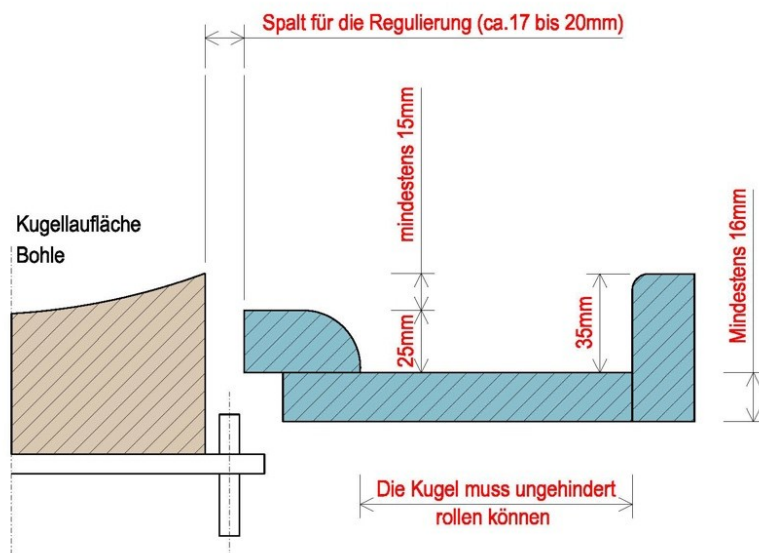
Abbildung 25 Beispiel für Ausführungen der Fehlwurfrinnen
