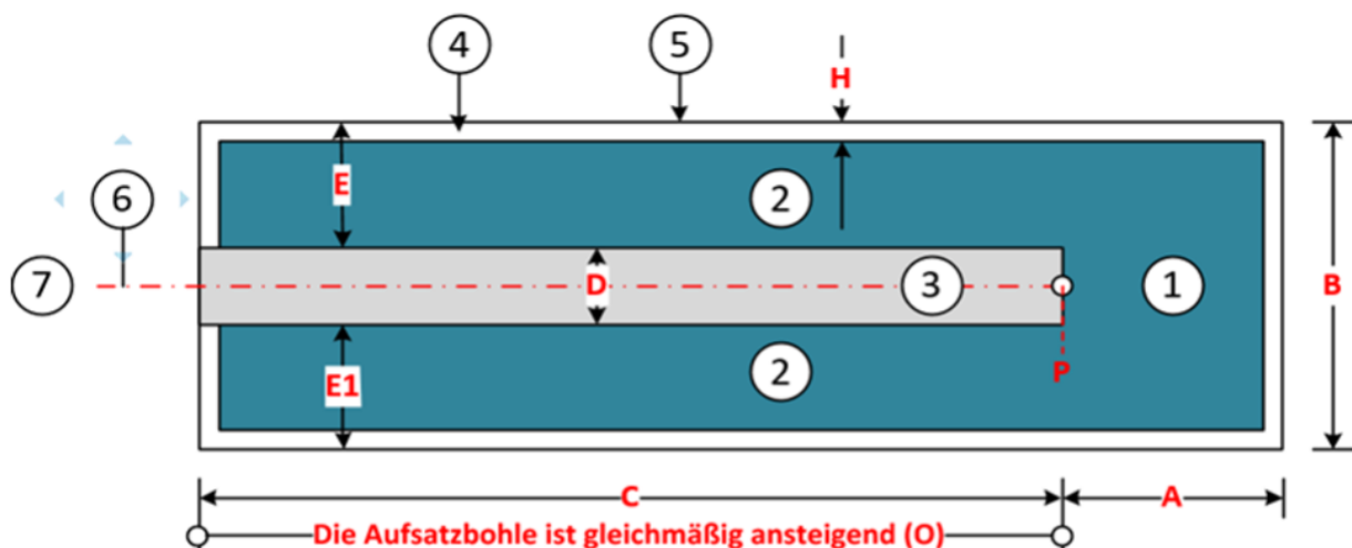
Abbildung 28 Der Spielbereich
